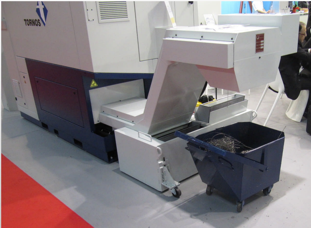
Convoyeur d'extraction des copeaux pour tour Tornos Sigma 20. Tapis métallique perforé, bac de décantation. Matière traitée: inox.
